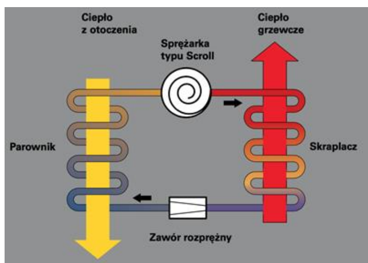
Rysunek 6: Obieg pompy ciepła
