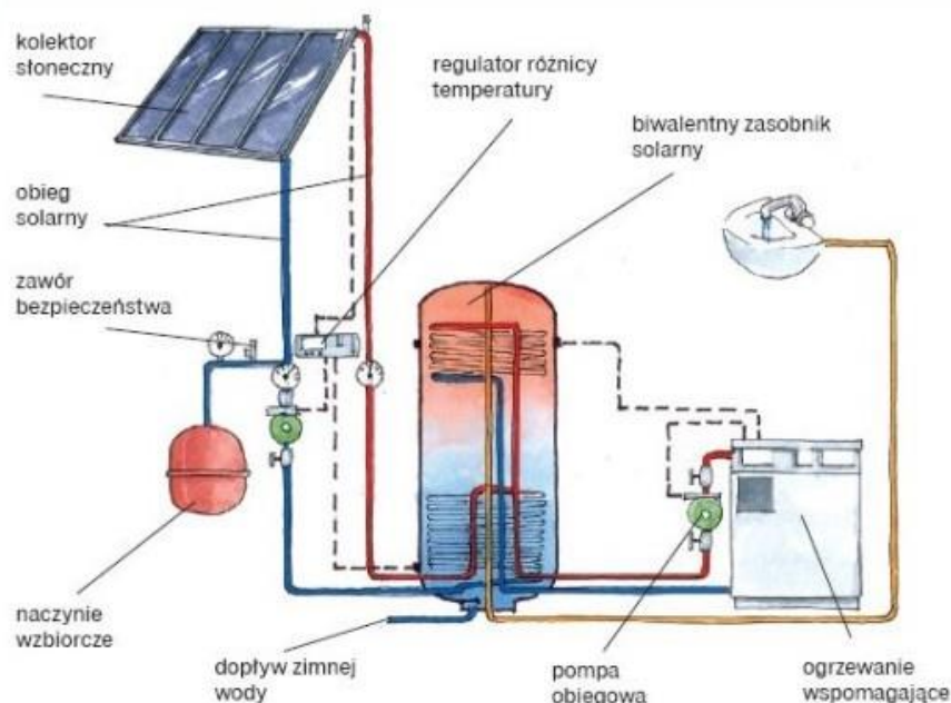
Rysunek 14: Schemat zasady działania kolektora słonecznego
