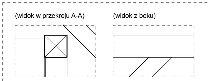
POŁĄCZENIE: płatew pośrednia - miecz
