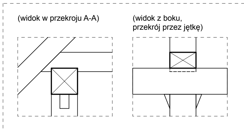
POŁĄCZENIE: krokiew - jętką - płatew pośrednia
